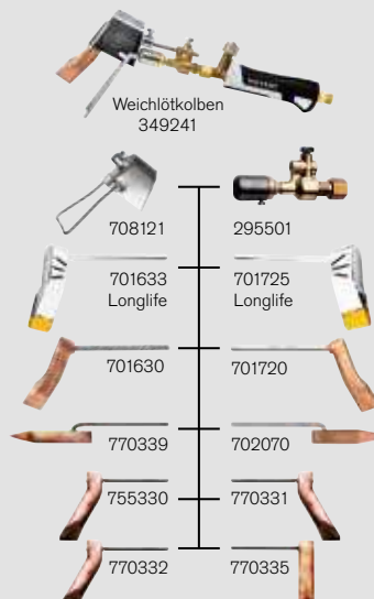
Kolbenlöten
