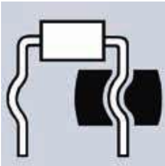
Zum Anbiegen eines Bogens als Spannungs-entlastung („stress relief“) / für Abstand zur Platine
