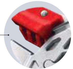
Kunststoff-Anlagebacke: schwenkbar für einen sauberen Bruch und optimalen Schutz der Fliese vor Beschädigungen
