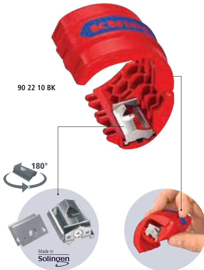
Der variable Messerblock lässt sich je nach Bedarf um 180 Grad gedreht einsetzen
