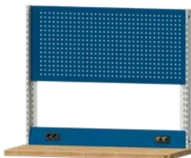
2 x Connect-Aufbaustütze H= 1200 mm; 1 x Lochwand H = 650 mm; 1 x Energiekanal mit 1 x Schuko-Doppelsteckdose 230 V/50 Hz, 10/16 A, 2-polig; 2 x Schnellkupplung Druckluft
