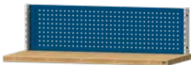
2 x Connect-Aufbaustütze H= 400 mm 1 x Lochwand H = 400 mm
