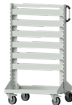
Grundwagen zusätzlich bestückt mit: 12 x Halteschiene 960.970 für Sichtlagerkästen
