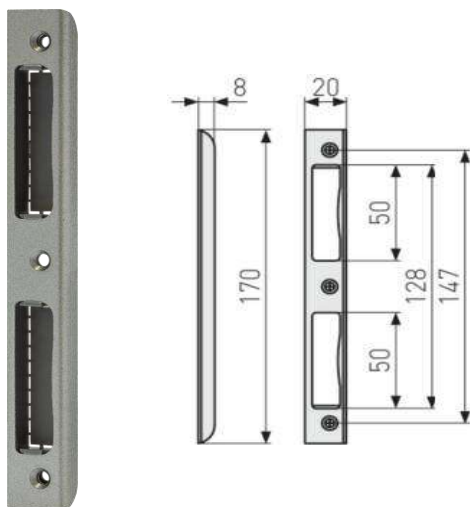
Schließblech für Innen- und Korridortüren " WSB 170 " Stahl - Schließblech mit Kunststoffeinlage silberfarbig
