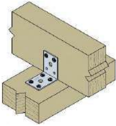
Winkelverbinder Stahl sendzimirverzinkt ohne Rippe
