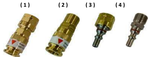
Sievert Schnellkupplungen & Kupplungsstifte
