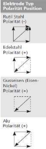
GYS Universal Stabelektroden in Kleinpaketten ( Blister ) Ausführungen für Stahl, Edelstahl, Guß und Aluminium
